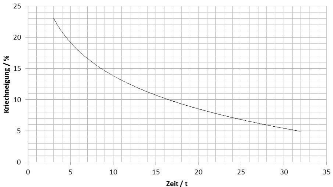
Diagramm 2: Mit dem Polyesterfaserschlauch "BRAWOLINER 3D" und dem Harzsystem "Combi-Tec® EP 60": Beurteilung der Kriechneigung in Abhängigkeit des Probenalters
