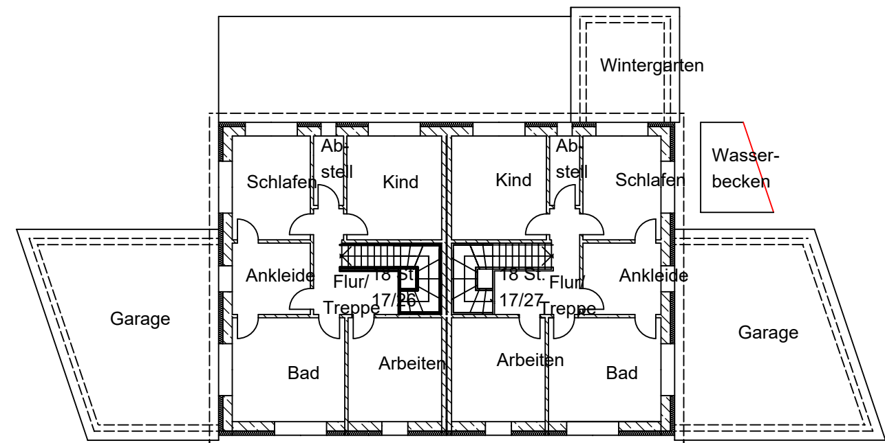
Obergeschoss M=1:200
