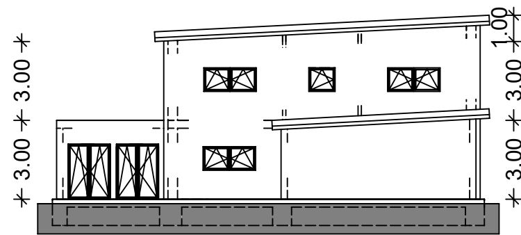
Seitenansichten M=1:200
