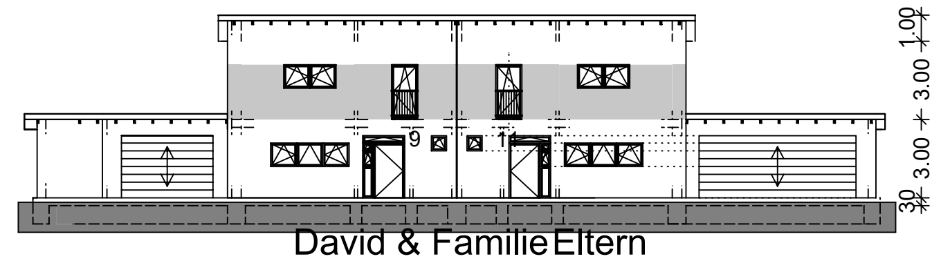
Straßenansicht M=1:200
