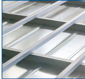
Bodenkonstruktion mit verzinktem Blindboden
