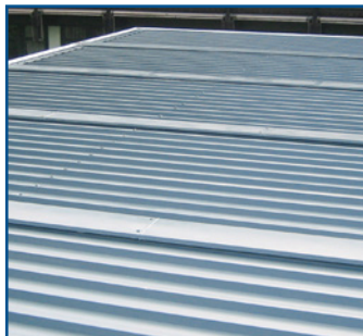
Dachkonstruktion aus verzinktem Blech und integrierter Regenwasserabführung
