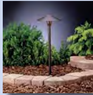
Weg-Lampe (IP54) mit rundem Schirm Gehäuse: Druckguss-Aluminium Leuchtmittel: 912X-Glühlampe, max. 24,4 W (Modell Nr. LP-W-15310-AZT)
